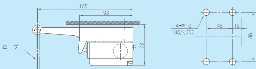
外形図 (mm)
