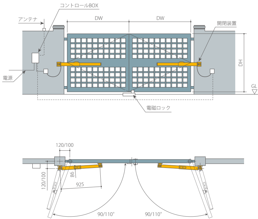
422型開閉装置
