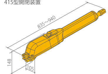
415型開閉装置
