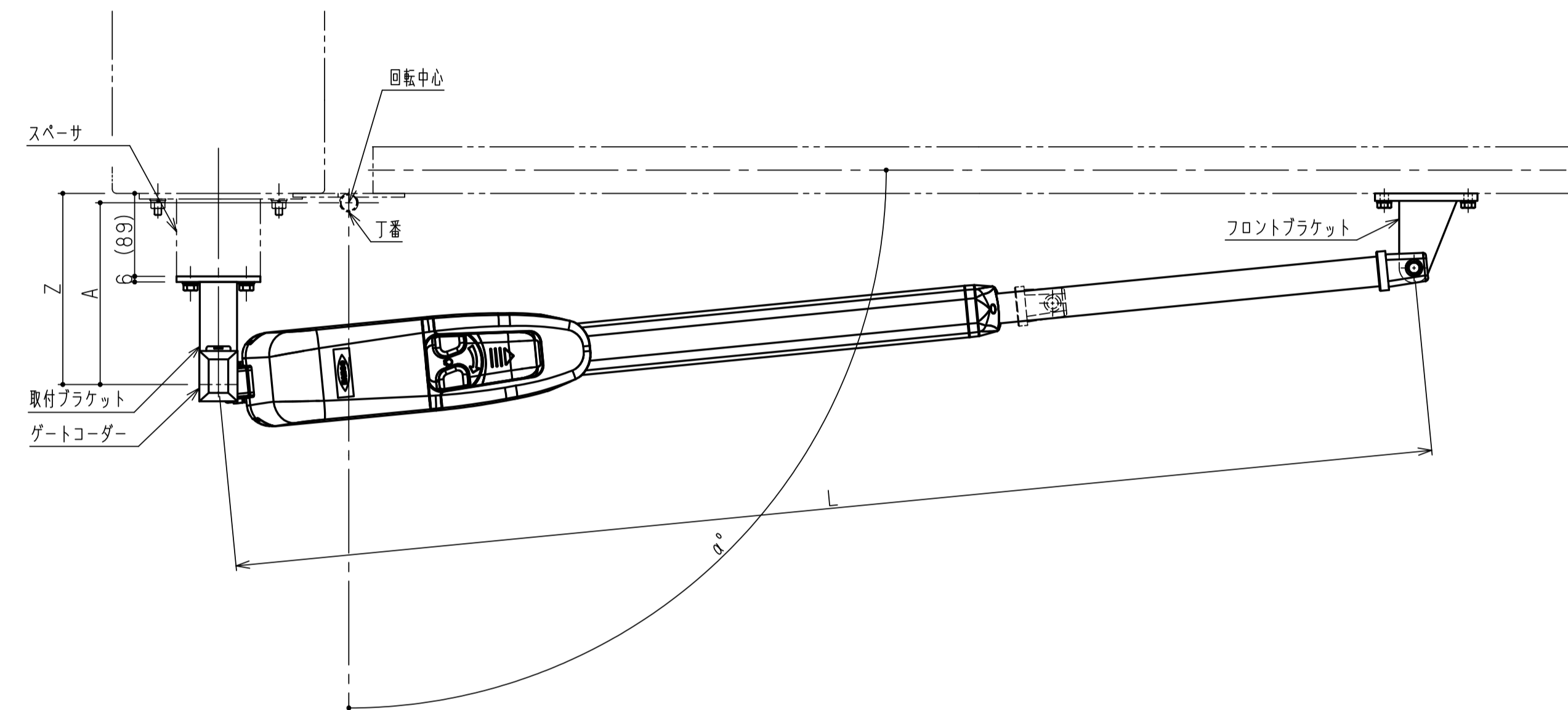
駆動部取付詳細 (1:5)
