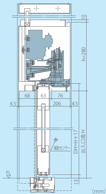
縦断面図
