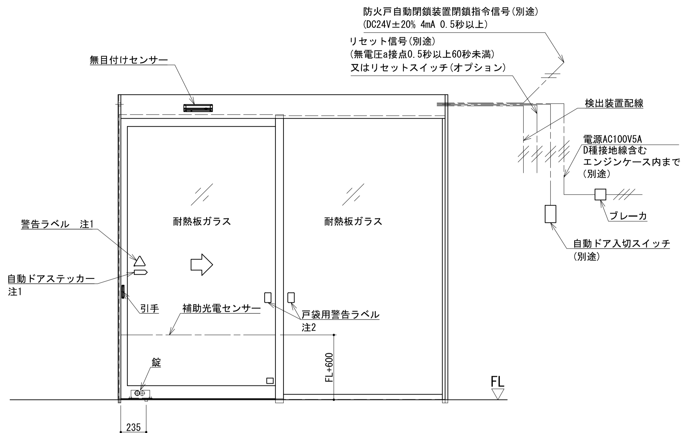
外観図(右勝手)
